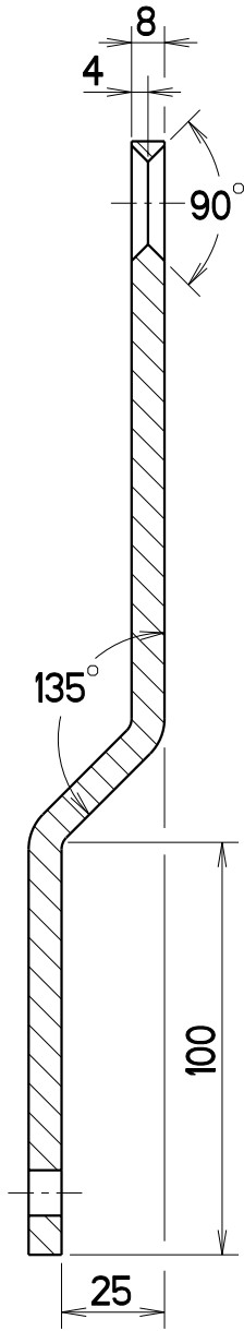
SECTION A-A
